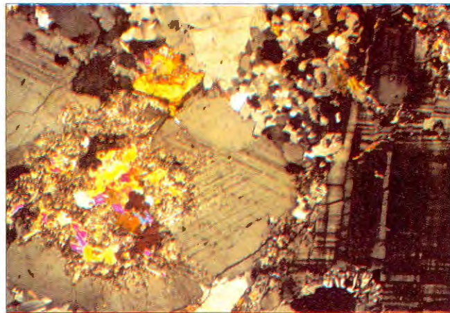
Figura 17. Granito migmatítico, a la izquierda se observa un cristal de plagioclasa, corroído por muscovita (en colores vivos), en medio de un mosaico de granos de cuarzo y a la derecha un fenoicristal de microclina.
