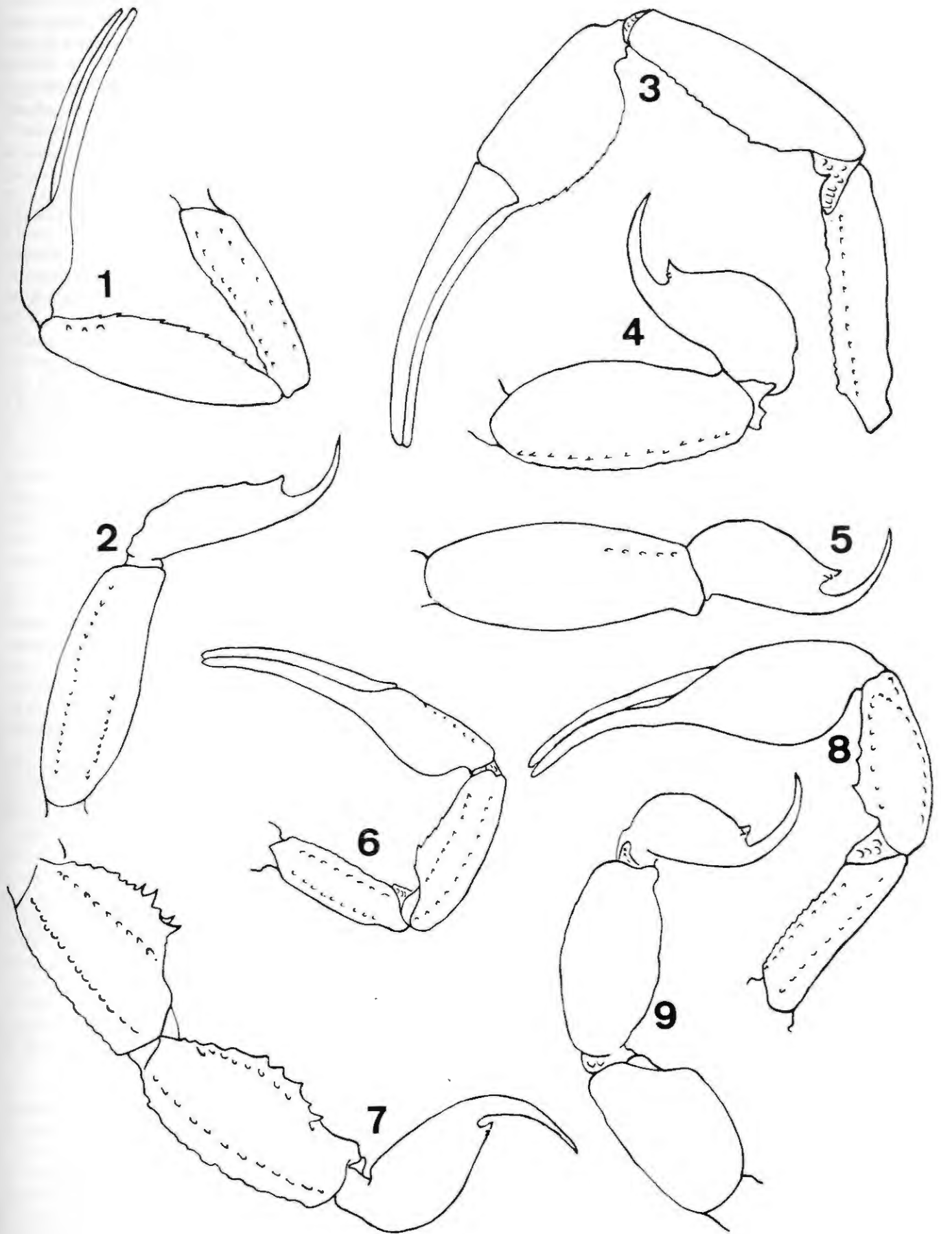
Figs. 1 et 2. Ananteris ehrlichi n.sp. (holotype-femelle): 1. Pédipalpe gauche, vue dorsale. 2. Anneau caudal V et telson, vue latérale. Figs. 3 à 5. Tiryus blanci n. sp. 3. Pédipalpe gauche, vue ventrale (holotype-mâle). 4. Anneau caudal V et telson, vue latérale (allotype-femelle). 5. Anneau caudal V et telson (holotype-mâle). Figs. 6 et 7. Tiryus cuellari n. sp. (holotype-femelle). 6. Pédipalpe droit, vue dorsale. 7. Anneaux caudaux IV et V et telson, vue latérale. Figs. 8 et 9. Tiryus sabineae n. sp. (holotype-mâle). 8. Pédipalpe droit, vue dorsale. 9. Anneaux caudaux IV et V et telson, vue latérale.
