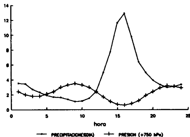
Figura 11. Comparación entre la variación diurna de la precipitación y la presión atmosférica en Bogotá.
