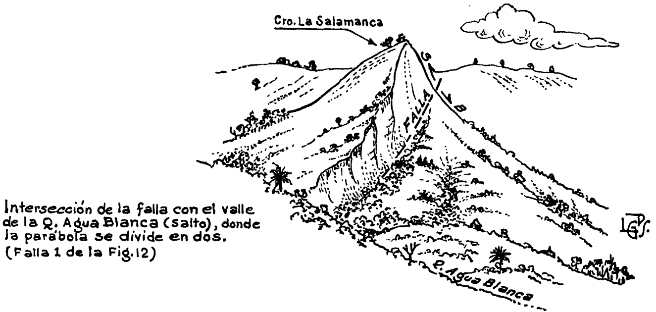
Fig. 11 - ALGUNOS ASPECTOS GEOMORFOLÓGICOS DE CORRIENTES ANALIZADAS
