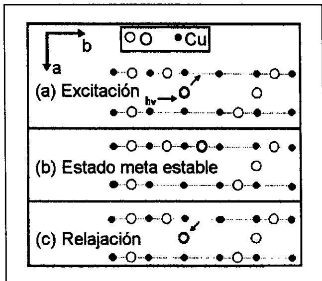
Figura 6. Mecanismo de ordenamiento de oxígeno fotoinducido: a) un fotón induce a un átomo de oxígeno a alargar la cadena de CuO_x , b) estado metaestable a bajas temperaturas ( T < 270 K), c) la relajación se da a temperatura ambiente y el oxígeno regresa a su posición inicial [11].
