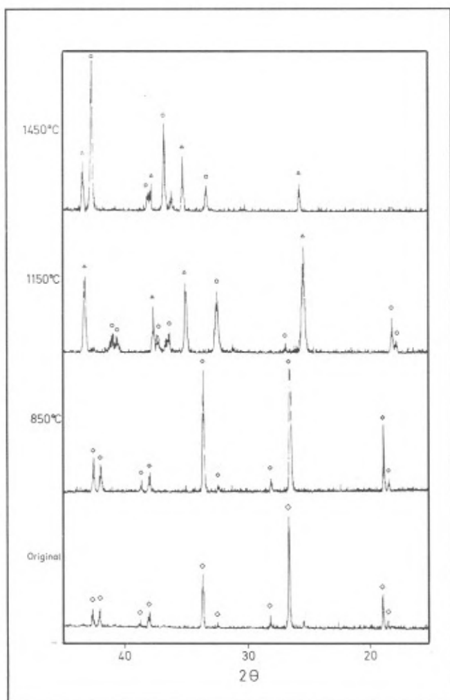
Figura 6. Espectros de difracción de rayos X (DRX) de un material de \beta\text{Al}_2\text{TiO}_5 tratado en atmósfera reductora ( 90\text{N}_2/10\text{H}_2 ) a temperaturas entre 850 y 1450° C. \beta\text{Al}_2\text{TiO}_5 = \text{AT} ; \text{Ps} = \text{Al}_{(2-2x)}\text{Ti}_{(1+2/3x)}\text{Ti}^{3+}_{(2/3x)}\text{O}_{(5-10/3x)} . ( \text{Ps}_1, x = 0 ), ( \text{Ps}_2, x = 1 )
