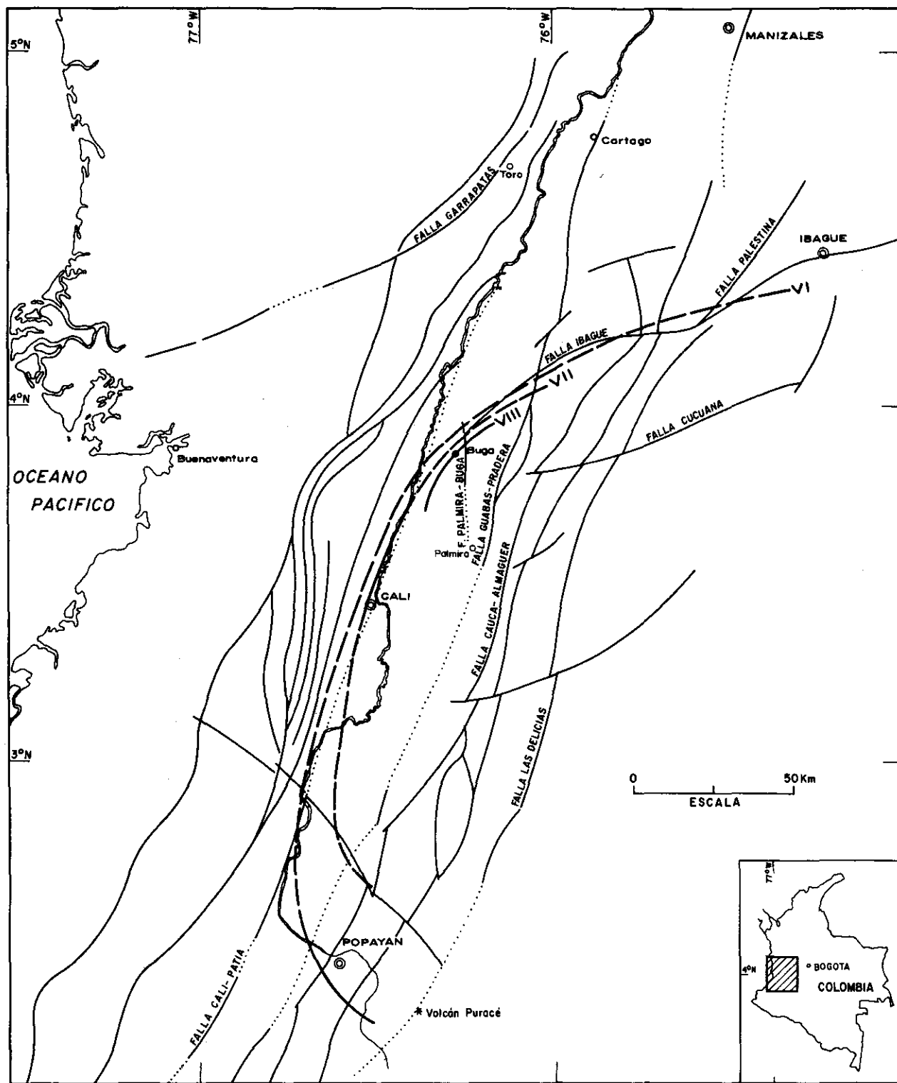
Figura 1. Isosistas y grandes fallamientos regionales en la zona de influencia del terremoto de Buga.
