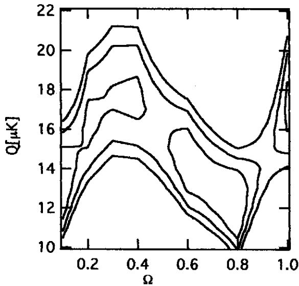
Figure 1: Contornos de igual probabilidad a 1, 2, y 3- \sigma para el likelihood de modelos con parámetro de densidad \Omega y normalización del espectro primordial Q .
