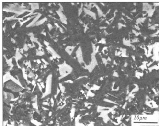
Figura 7. Microestructura por MEB de un material compuesto de \text{Al}_2\text{O}_3 - \text{TiO}_2 obtenido por reacción eutectoide de \text{Al}_2\text{TiO}_5 tratado térmicamente a 1150^\circ\text{C} durante 90h.
