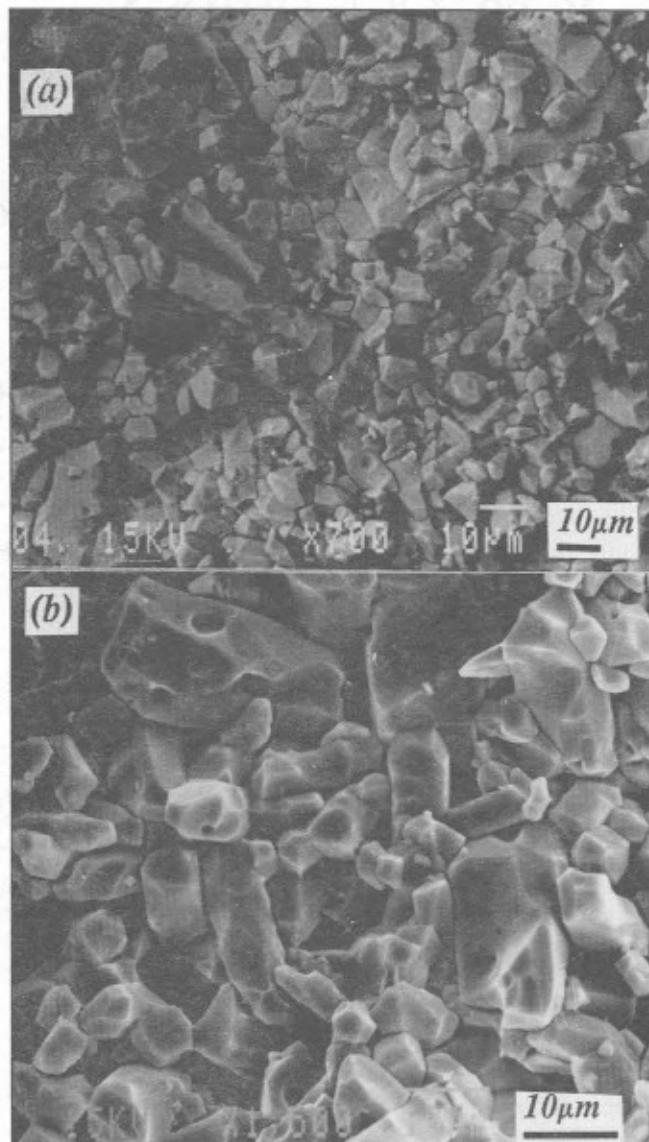
Figura 5. Microfotografías típicas obtenidas por MEB de superficies de fractura de la muestra MAT donde se aprecia la morfología de los granos de \beta Al_{2(1+0.3)}Mg_{0.12\pm 0.05}Ti_{(1\pm 0.02)}O_{(5\pm 0.2)} a distintos aumentos.
