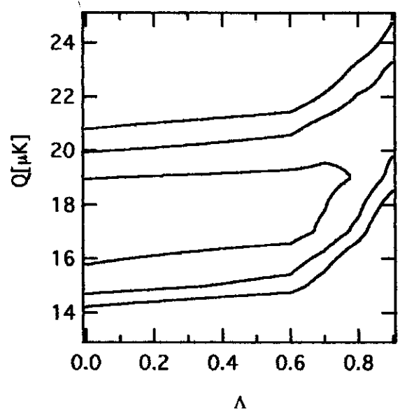
Figure 2: Contornos de igual probabilidad a 1, 2, y 3- \sigma para el likelihood de modelos con constante cosmológica \Lambda y normalización del espectro primordial Q .
