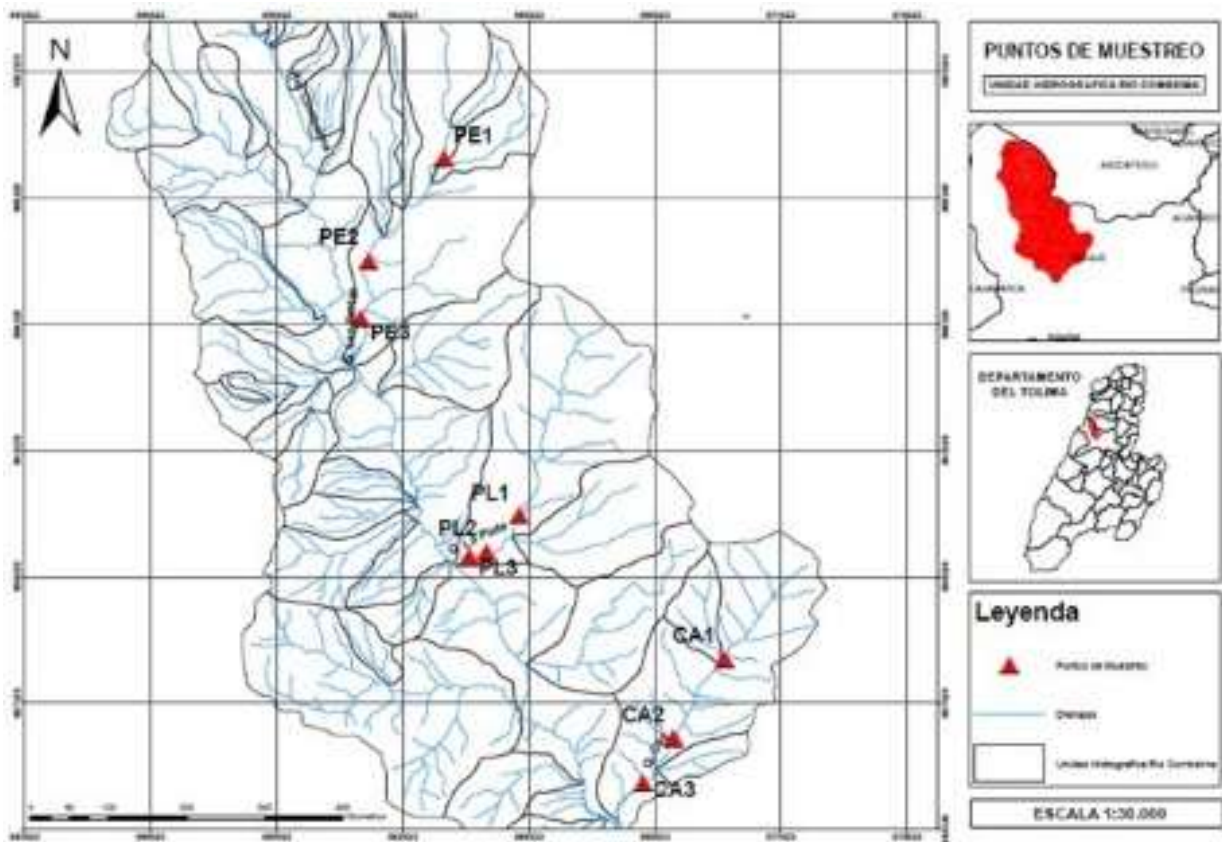
Figura 1S. Mapa de la cuenca del río Combeima y puntos de muestreo
