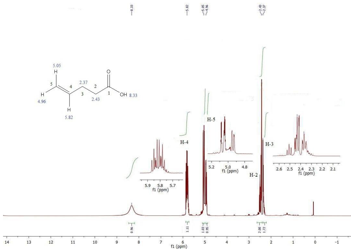
Figura 5S. Espectro MS del compuesto I
