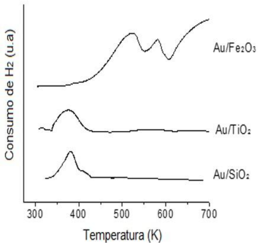
Figura S2. Comportamiento de reducción de los catalizadores de oro soportado (TPR-H 2 ).
