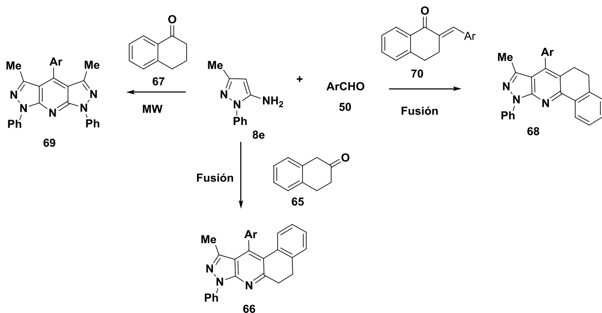
Figura 16S. Síntesis de benzopirazoloquinolinas.
