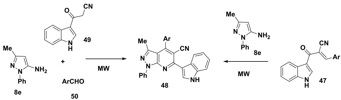
Figura 12S. Síntesis de indolipirazolo[3,4- b ]piridinas.
