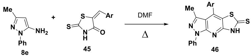
Figura 11S. Síntesis de tiazolopirazolopiridinas.
