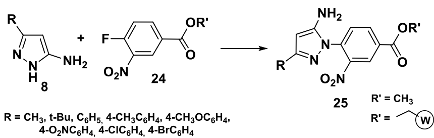
Figura 7S. Modificación de aminopirazoles en fase sólida.
