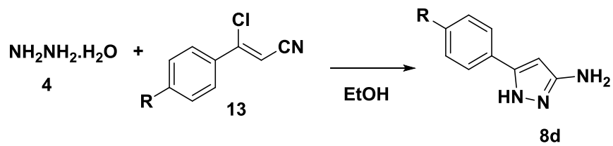
Figura 3S Síntesis de aminopirazoles a partir de \beta -clorocinamonitrilos.
