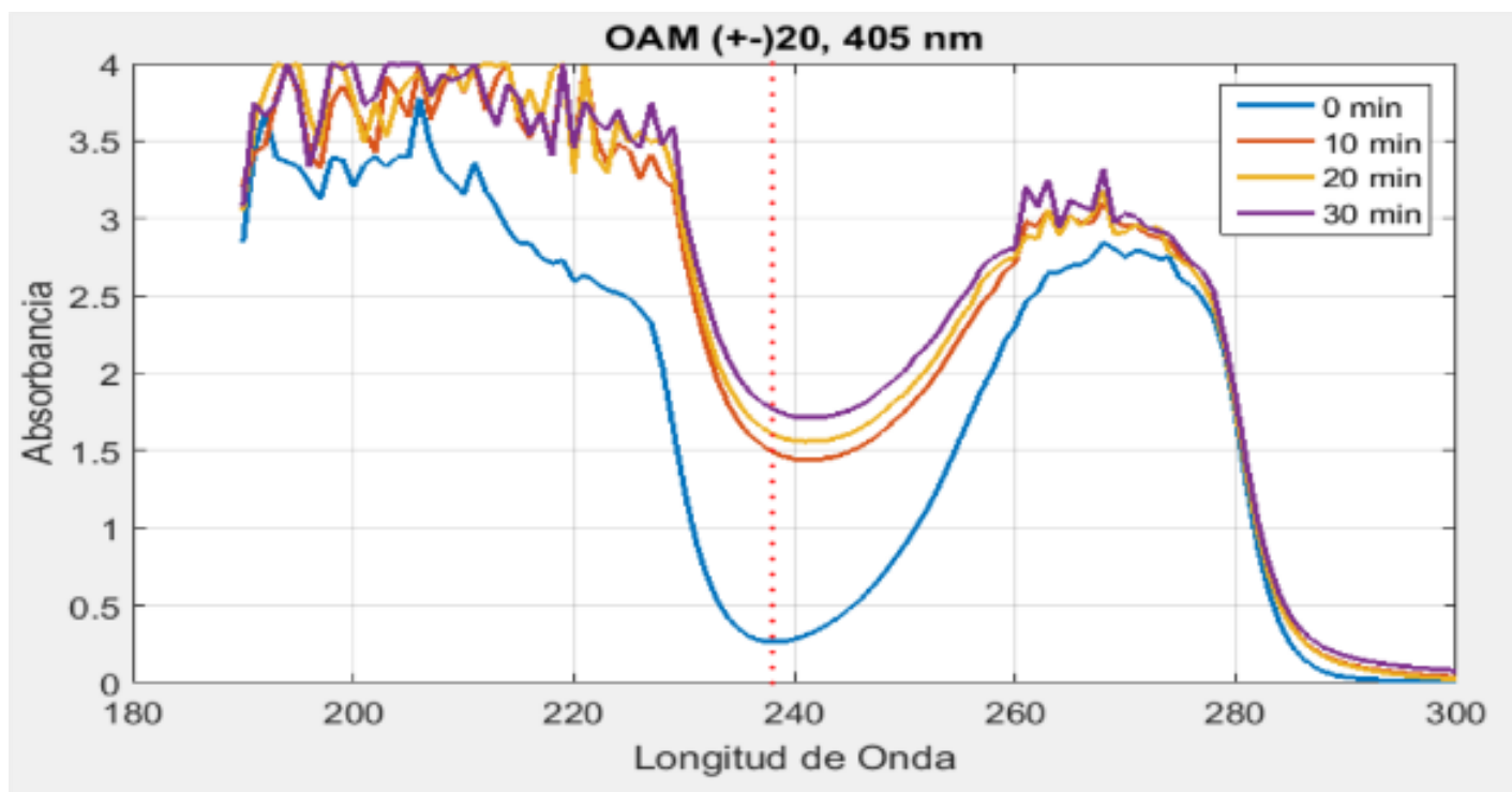
Figura 9S. Absorbancia de la reacción irradiada con un haz de 405 nm, catalizador NTiO 2 y superposición de cargas topológicas opuestas \pm 20 . Fuente autores.
