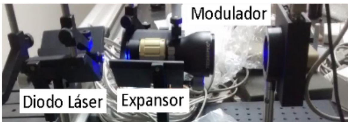
Figura 2S. Montaje experimental. Fuente autores a y b.
