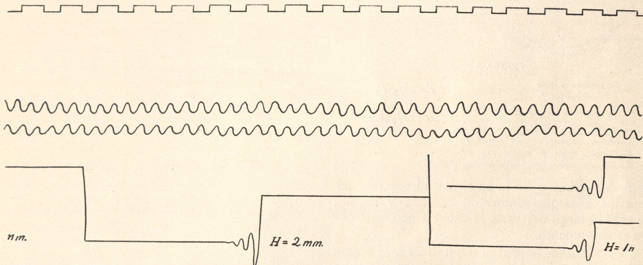
Gráfica de las oscilaciones de la columna manométrica en un aparato inscriptor.
