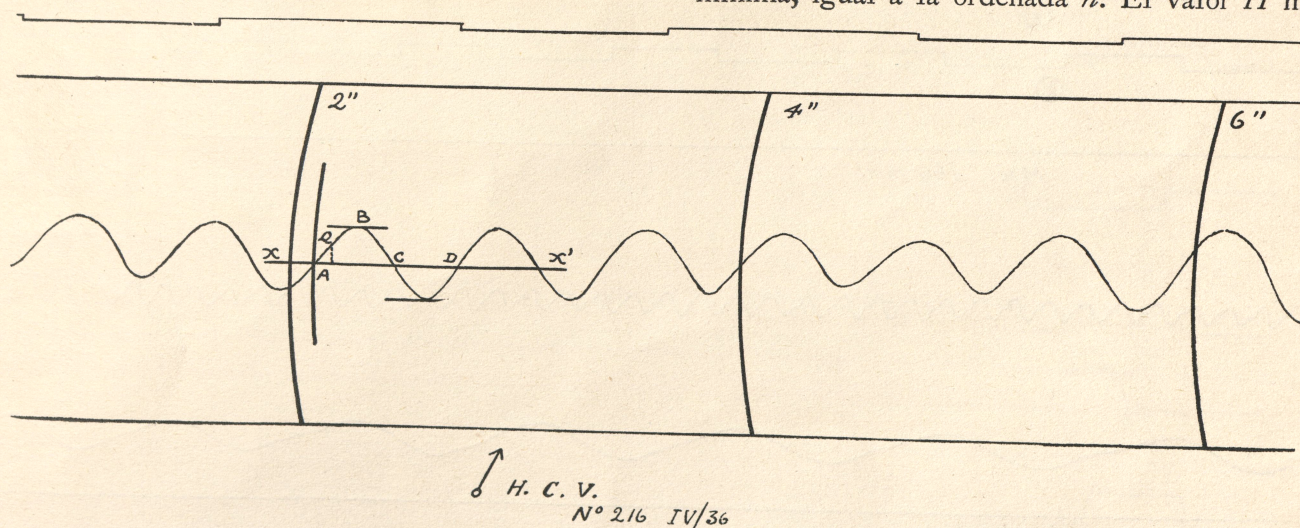
Curva del movimiento ondulatorio a lo largo de una arteria.
