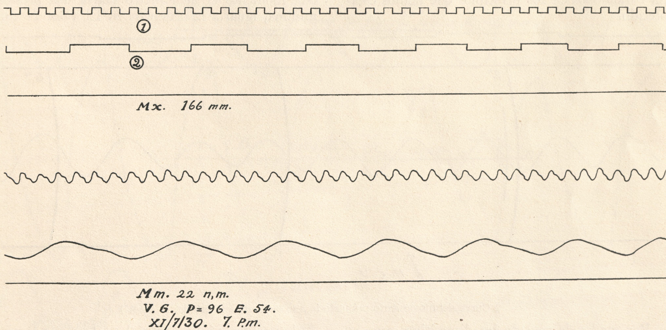
Gráfica de las oscilaciones de la columna manométrica en un aparato inscriptor.
