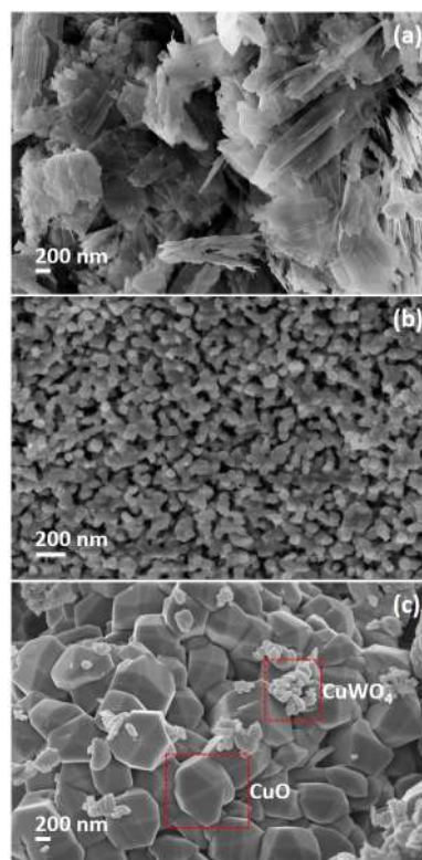
Figura 4. Imágenes obtenidas con microscopía electrónica de barrido con emisión de campo de (a) CuO (Mag = 50,00 KX), (b) CuWO 4 (Mag = 100,00 KX) y (c) CuO/CuWO 4 (Mag = 50,00 KX). En los tres casos la barra de guía es de 200 nm. Fuente: elaboración propia
