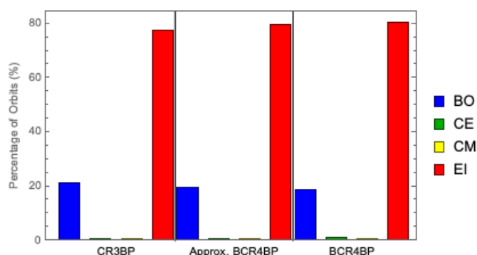
Figura 8. (Color en línea). Porcentaje de órbitas para la clasificación orbital en el plano (x, J) en las cercanías de los cuerpos primarios, mostrada en la Fig. 5. El código de colores y la disposición de los paneles son los mismos que en la Fig. 7.
