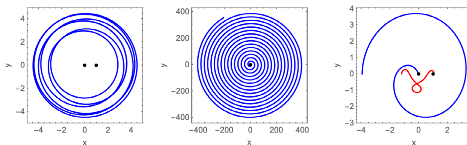
Figura 3. (Color en línea). Órbitas representativas en el plano (x, y) : movimiento acotado (izquierda), escape al infinito (centro) y colisión con los primarios (derecha). La figura resalta las posiciones de los primarios (Tierra y Luna), indicadas por puntos negros en x_1 = -\mu y x_2 = 1 - \mu , respectivamente.
