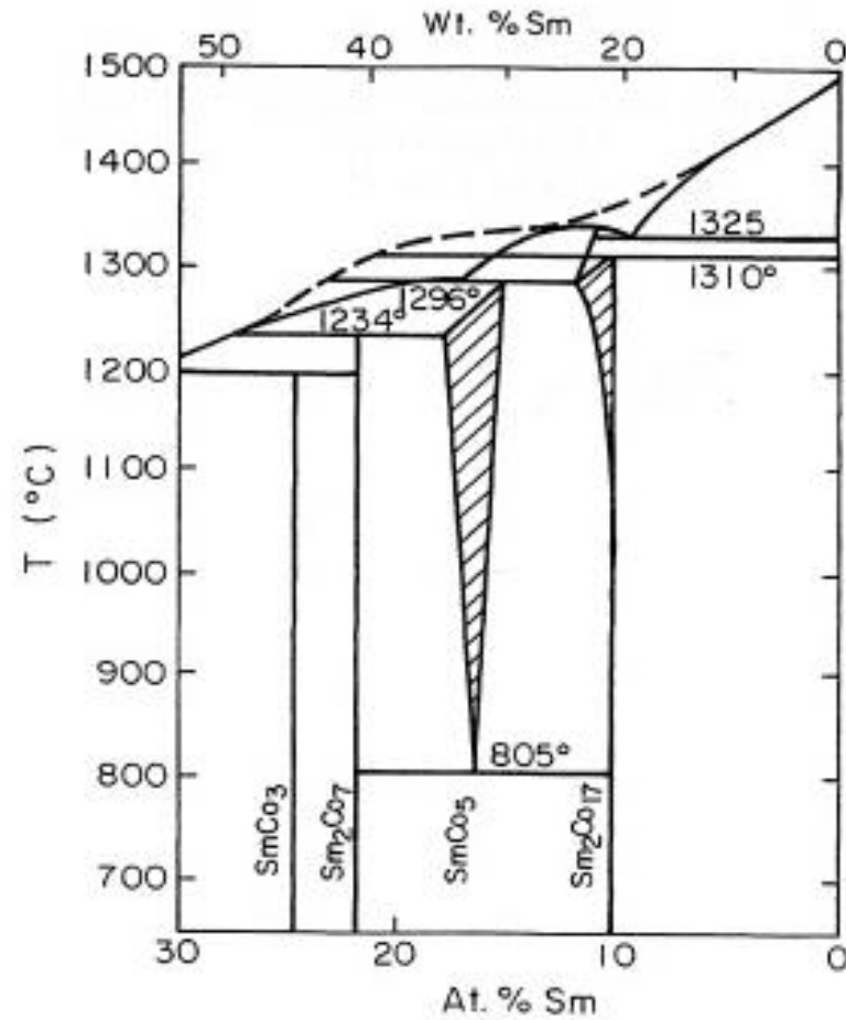
Figura 16S. Diagrama de fase de equilibrio del sistema SmCo en la región rica en Co ( Den Broder & Buschow (1977) ).
