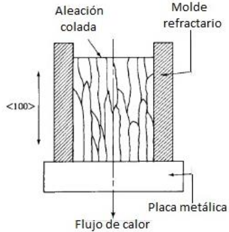
Figura 12S. Solidificación direccional de alnico a lo largo de [100] .
