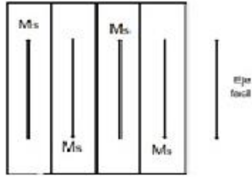
Figura 8S. Estructura de dominios de un sistema uniaxial.
