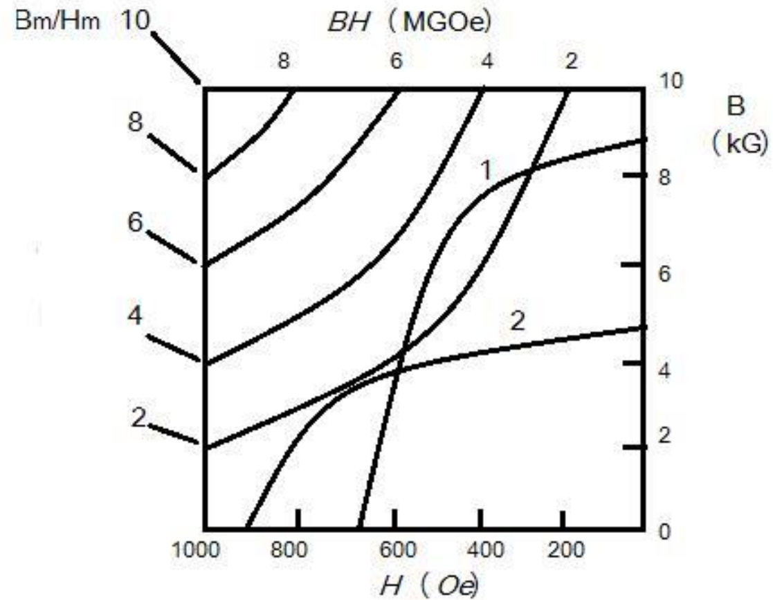
Figura 4S. Curvas de desmagnetización de los imanes 1 y 2, junto con diferentes curvas de BH constante y pendientes o permeabilidades.
