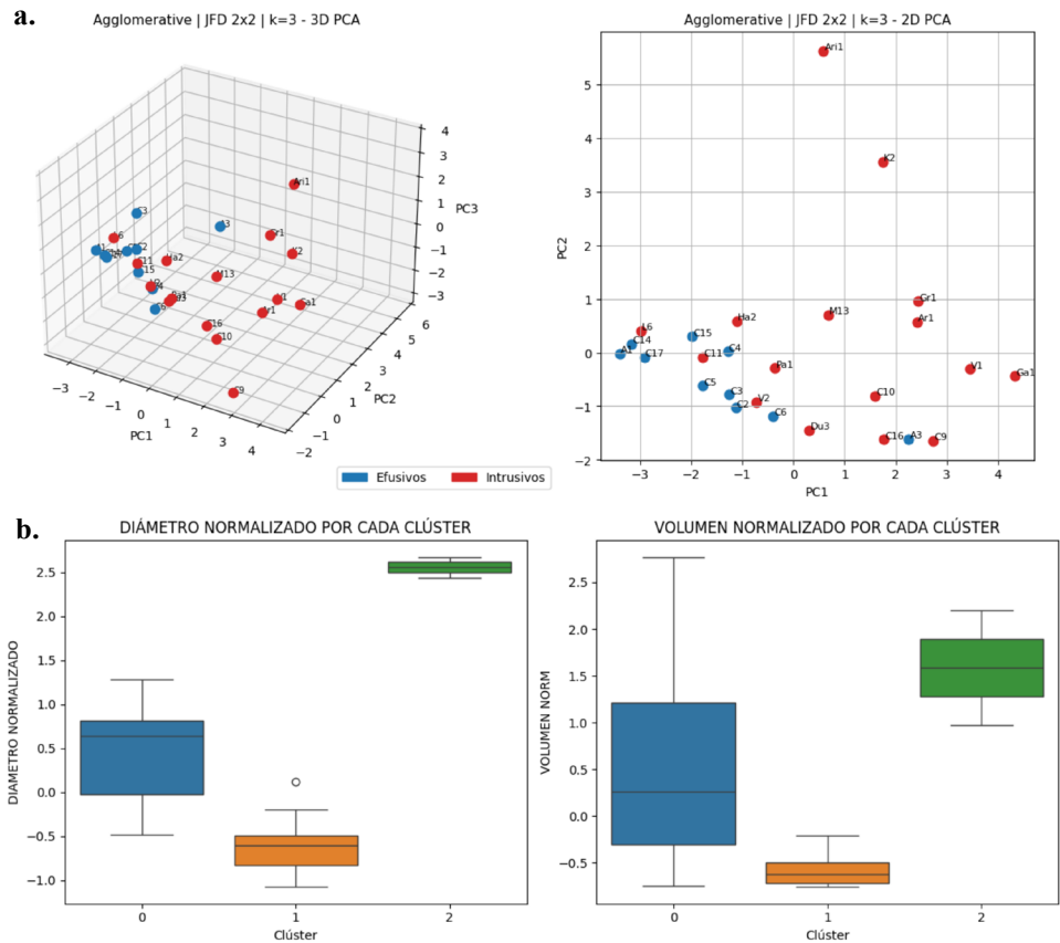
Figura 5. a. Agrupamiento Agglomerativo | JFD 2x2 | k=3, con etiquetas por tipo (efusivo/intrusivo). b. Diagramas de caja (boxplots) con las distribuciones del diámetro y el volumen normalizados para cada grupo obtenido en el mejor resultado de agrupamiento (Agglomerative | JFD 2x2 | k = 3). Los clústeres corresponden al grupo 0 (domos intrusivos clásicos), el grupo 1 (domos efusivos compactos) y el grupo 2 (domos intrusivos masivos).
