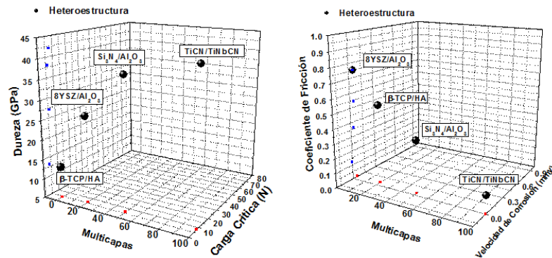
Figura 7. Índices de mérito para las heteroestructuras de [TiCN/TiNbCN] 200 , [Si 3 N 4 /Al 2 O 3 ] 70 , [8YSZ/Al 2 O 3 ] 70 y [β-TCP/HA] 50 depositadas sobre aceros industriales en función de los materiales y el número de capas. (a) Índice que relaciona dureza, carga crítica de desgaste y número de capas (n), y (b) coeficiente de fricción, velocidad de corrosión y número de capas (n) de las multicapas
