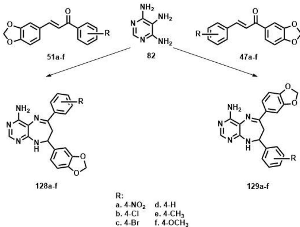
Figura 30S. Síntesis de nuevas 4-amino-6-aryl-8-(1,3-benzodioxol-5-il)-8,9-dihidro-7H-pirimido [4,5- b ][1,4] diazepinas 128a-f y 4-amino-8-aryl-6-(1,3-benzodioxol-5-il)-8,9-dihidro-7H-pirimido[4,5- b ][1,4]diazepinas racémicas 129a-f .
