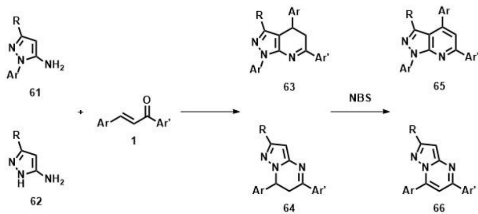
Figura 19S. Condensación de aminopirazoles NH -sustituidos 61 y NH -no sustituidos 62 con chalconas 1 y posterior aromatización de los productos con NBS.
