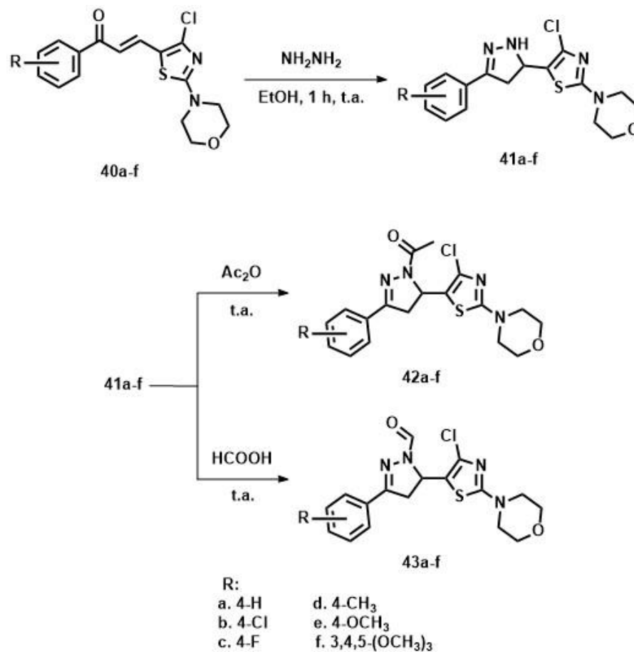
Figura 12S. Obtención de los compuestos 41a-f y posterior tratamiento con anhídrido acético o ácido fórmico.
