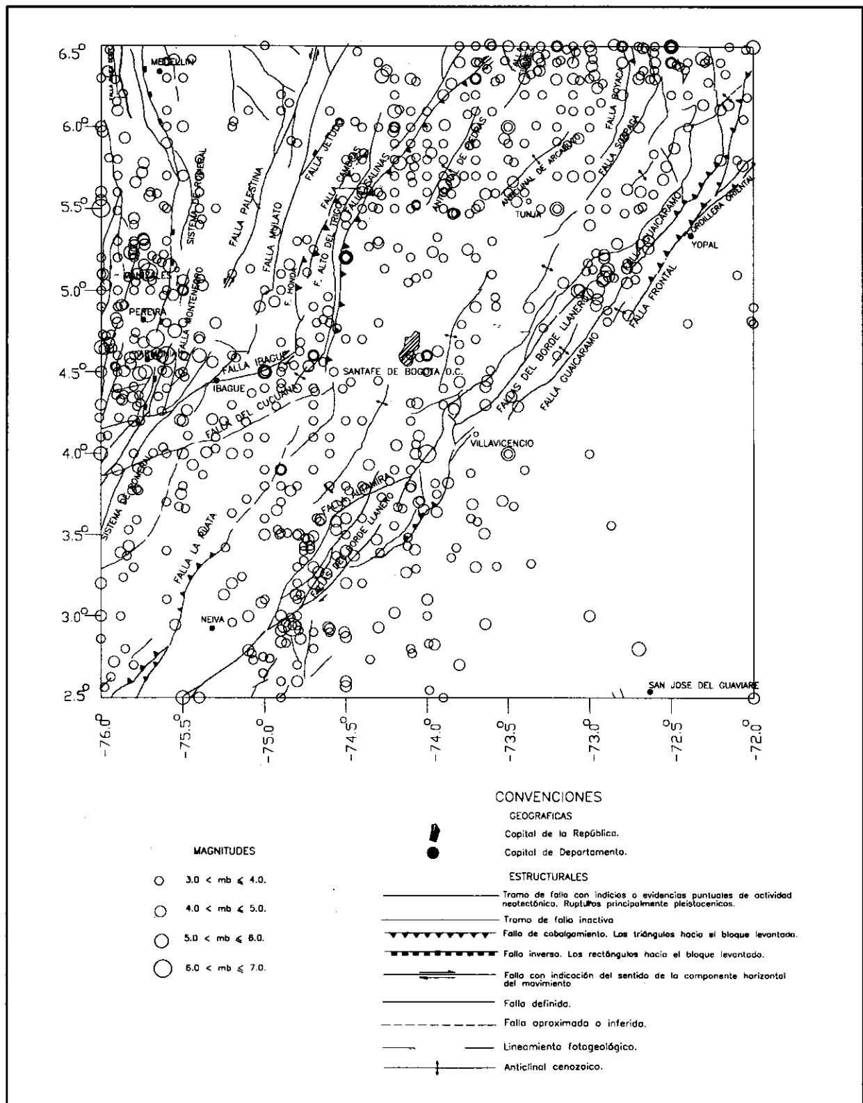
Figura 2. Sismicidad de la Región Central de Colombia, correspondiente al período entre 1900 y 1995, para sismos con magnitud m_b > 3.0 .
