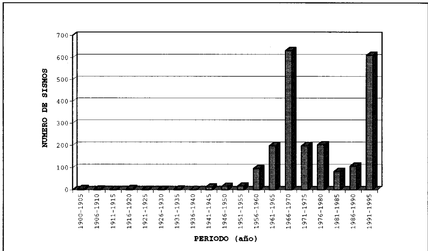
Figura 3. Distribución del número de sismos con el tiempo, para eventos con m_s > 3,0 ocurridos entre 1900 y 1995. Llama la atención la presencia de los picos en los períodos de 1966-1970 y 1991-1995.
