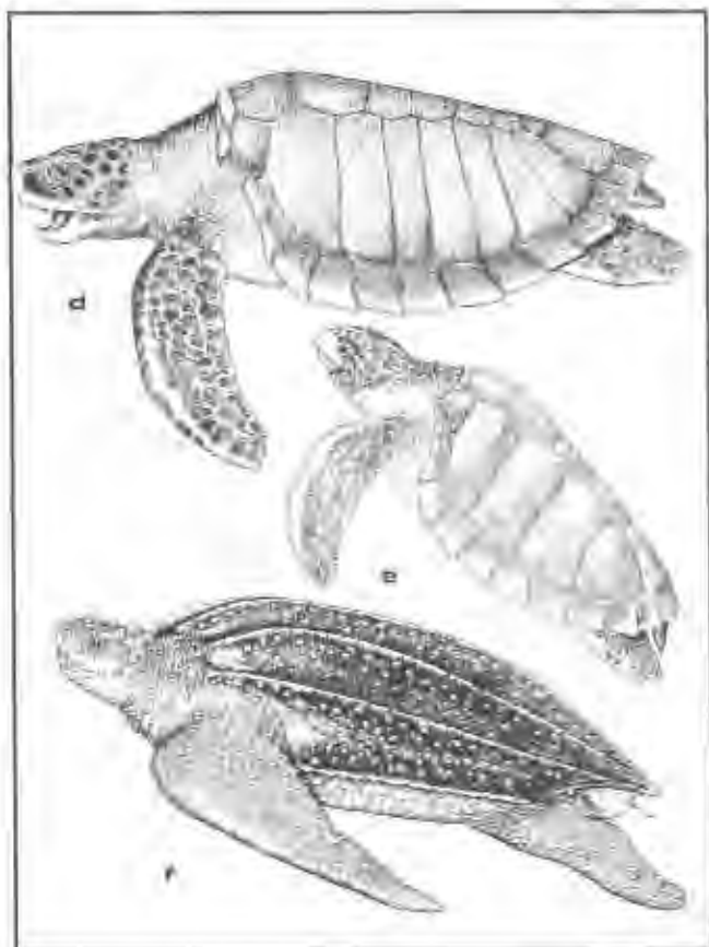
Fig. 2. Tortugas de Colombia: (a) Lepidochelys kempi (Garman, 1880), (b) Lepidochelys olivacea (Eschscholtz, 1829), y (c) Dermochelys coriacea coriacea (Nardo, 1761); ilustraciones por gentileza de la FAO.
