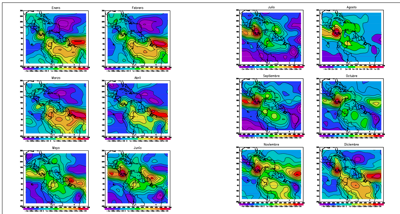
Figura 7. Ciclo anual promedio de la divergencia del viento horizontal [1/s] por 200 hPa, sobre el trópico Americano. Fuente de datos: Reanálisis Climático NCEP/NCAR para el período 1958-1998.
