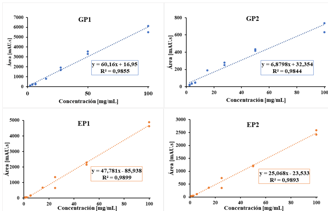
Figura S3. Curvas de calibración. La figura muestra las curvas de calibración para los picos detectados en los cromatogramas de los extractos glicólico y etanólico de C. spinosa . GP1: pico 1 en el extracto glicólico; GP2: pico 2 del extracto glicólico; EP1: pico 1 del extracto etanólico y EP2: pico 2 del extracto etanólico.
